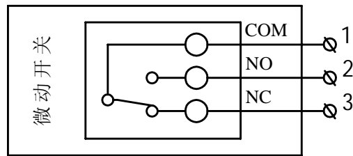
微动开关原理图
